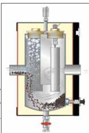
Trio Schnittbild
